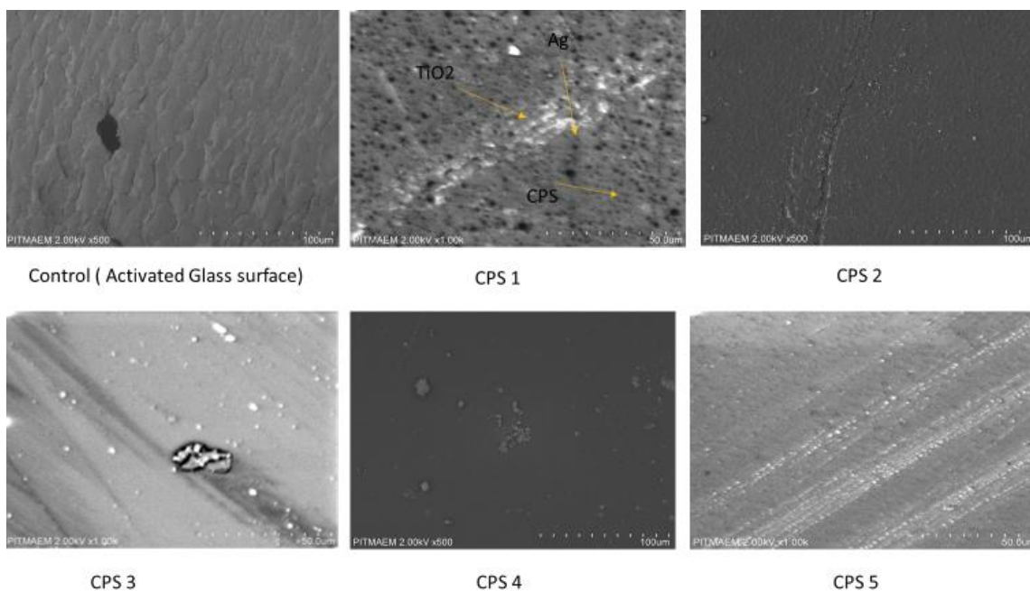
Fig. 19: SEM analysis.
